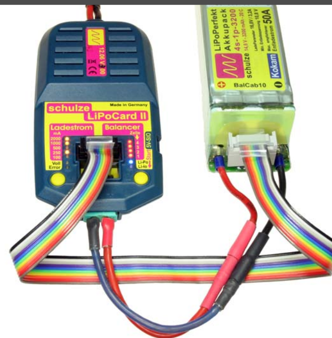
Schulze LiPoCard2 mit dem Schulze LiPoPerfekt Akkupack verbunden über das Schulze BalCab10-Verlängerungskabel .
