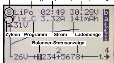
Bild 7.7, Kurvenbildschirm Akku1
