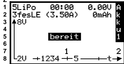
Z Bild 23.8.A1 Kurven-Bildschirm Akku1
