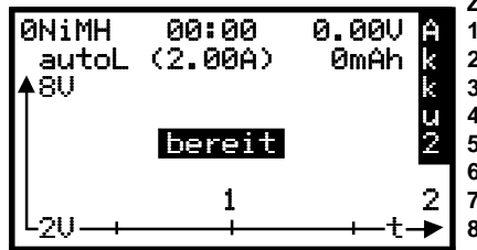
Kurven-Bildschirm Akku2 Bild 23.8.A2 Z
