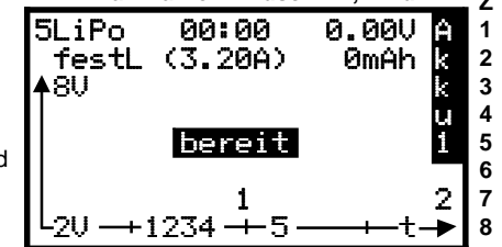
Akku1 Kurven-Bildschirm, Bild 7.2.1 Z
